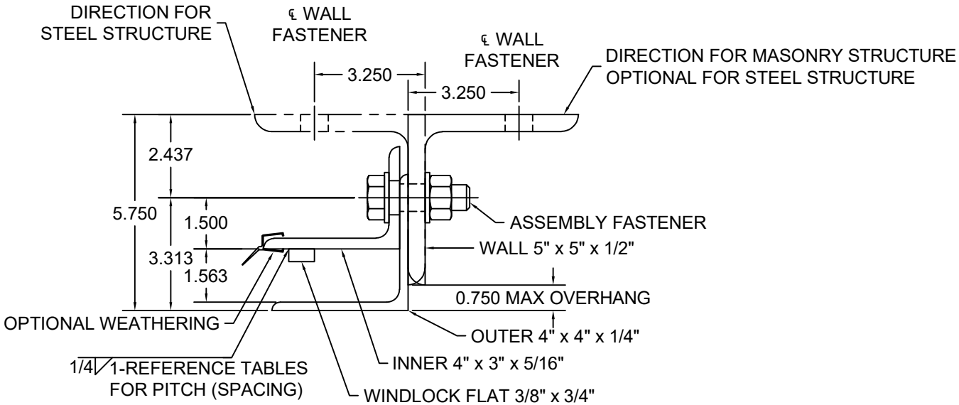
GUIDE ASSEMBLY TYPE 548 SCALE: 3" = 1'-0"
