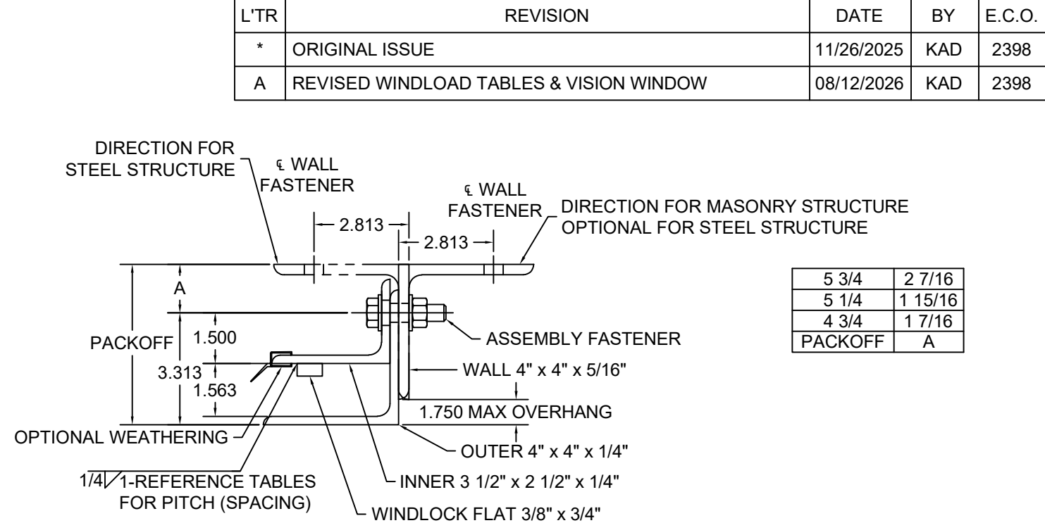
GUIDE ASSEMBLY TYPE 445 SCALE: 3" = 1'-0"
