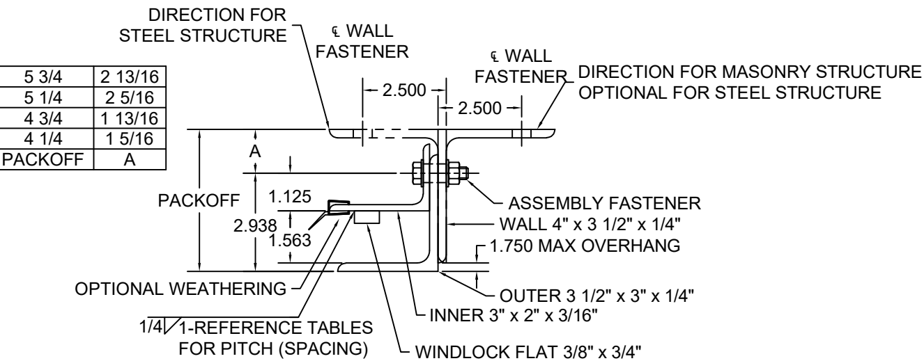
GUIDE ASSEMBLY TYPE 344 SCALE: 3" = 1'-0"
